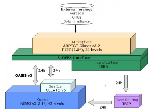
Illustration 2: Représentation des différentes composantes du modèle CNRM-CM5
