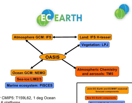
Illustration 2: Représentation des différentes composantes du modèle EC-EARTH
